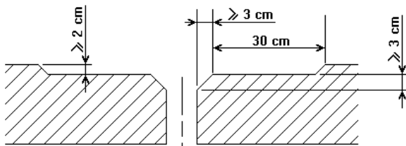
Figure 9 – Feuilleure pour étanchéité asphalté
