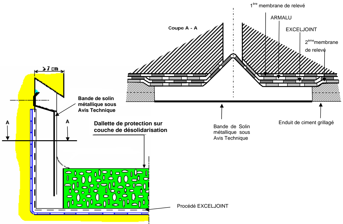
Figure 25 – Exemple de protection en tête de relevé
