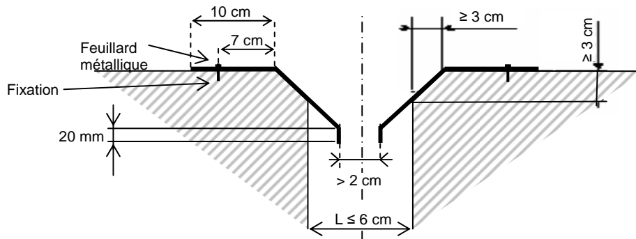
Figure 8 – Joint en zone de sismicité non nulle
