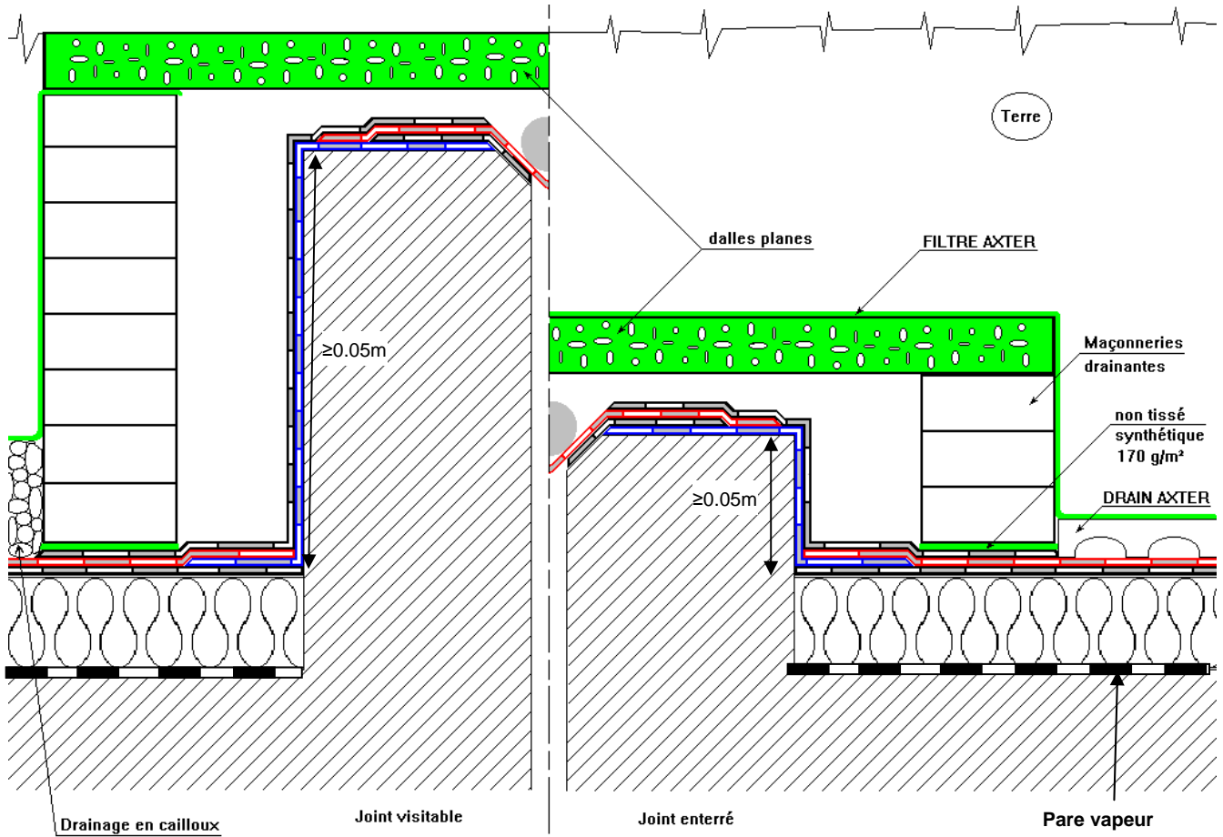
Figure 26 – Exemple de protection de joint de terrasse-jardin
